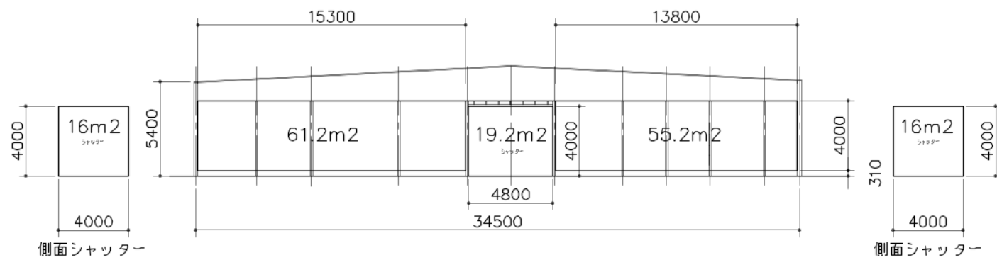
吸気側断面図
