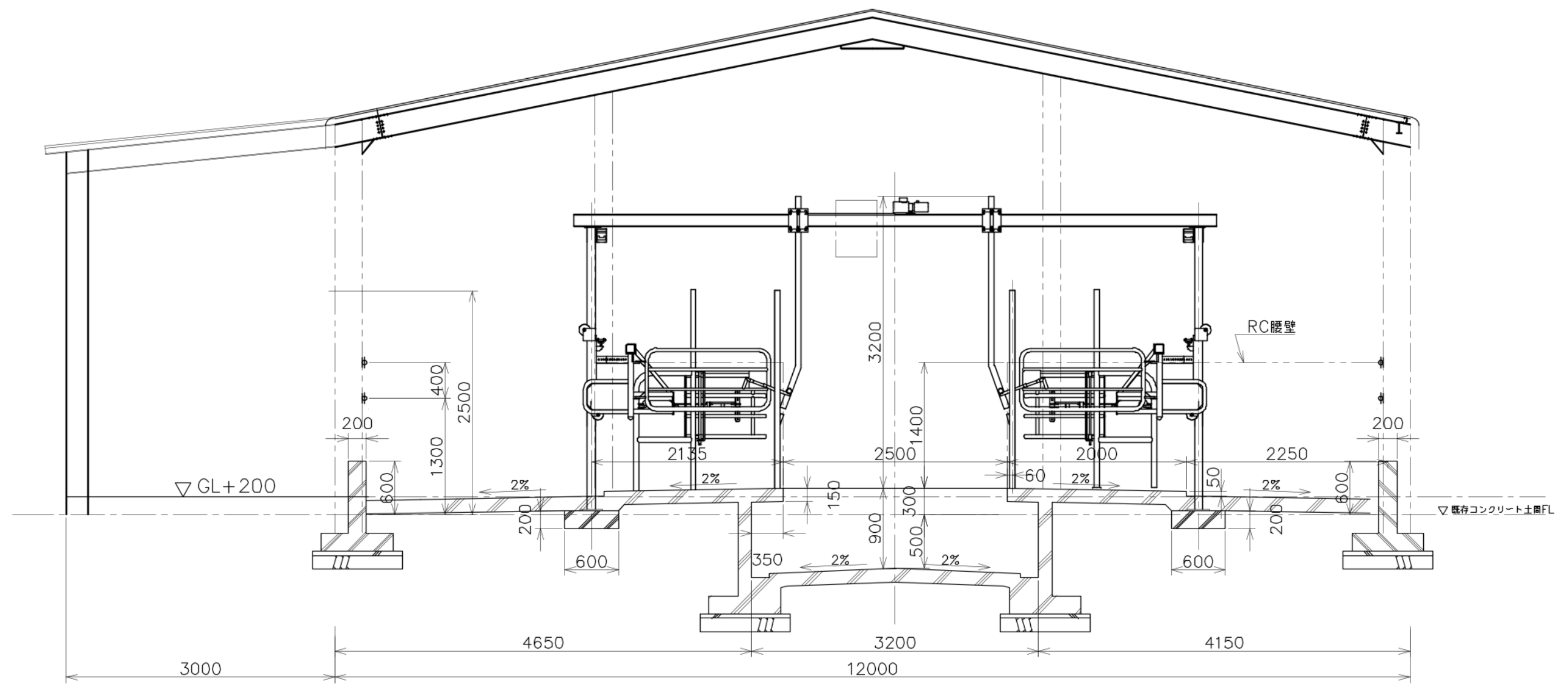
搾乳ピット断面図
