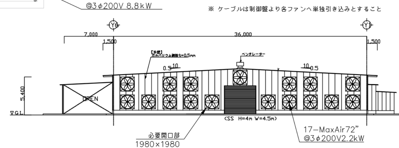
西側立面図 S:1/200
