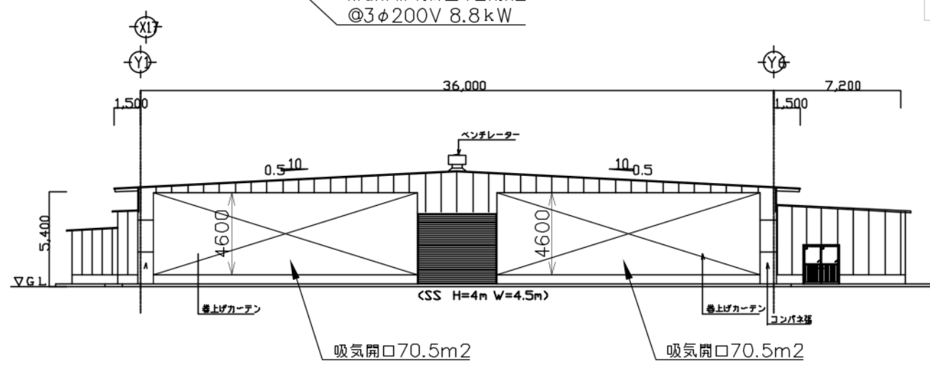
東側立面図 S:1/200
