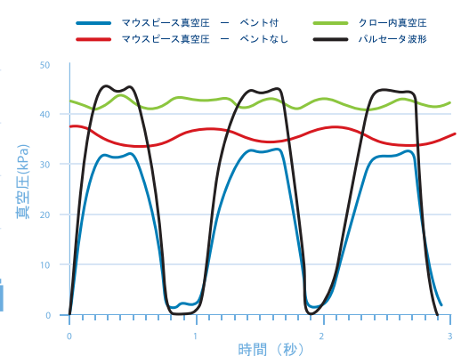
搾乳終了間際のパルセーションと真空変動
